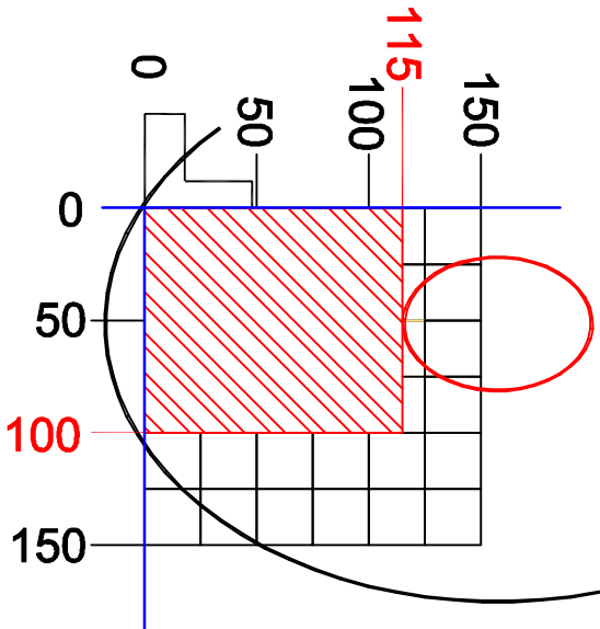
45° : 100 x 115 mm
